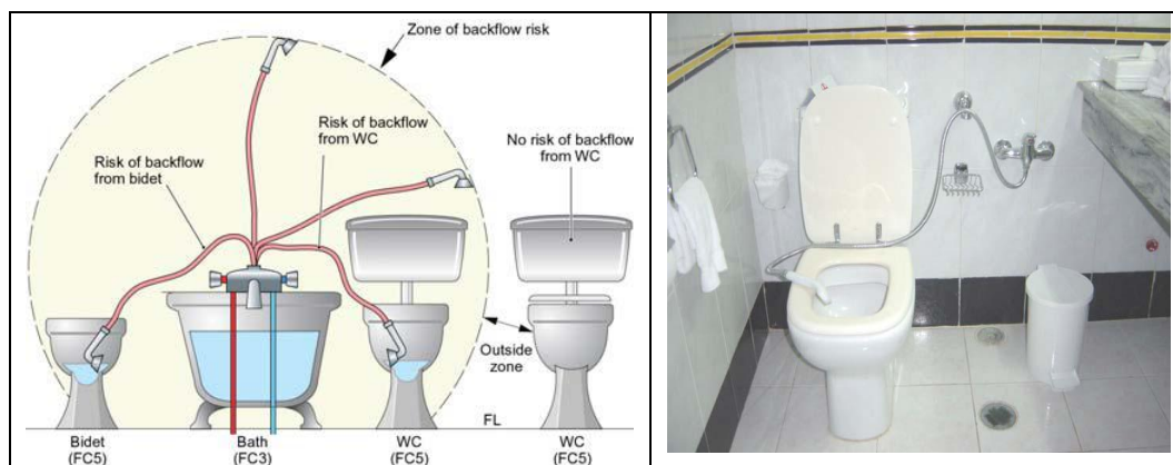
Figur 2.5 Eksempel på mulig tilbagesugning fra forskellige typer af installationsgenstande
